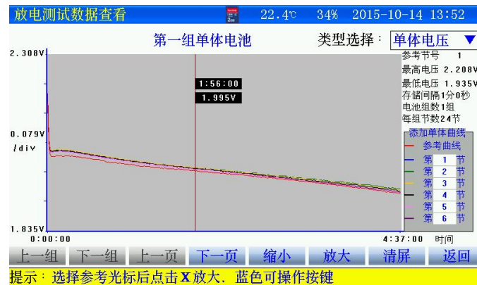
图 3.7.4-1 单体电压曲线界面
