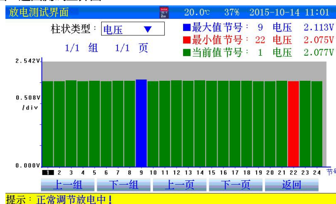
图 3.2.4-1 单体电压柱状图
