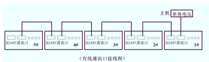
图 2.4.4.4 有线通讯口接口图
