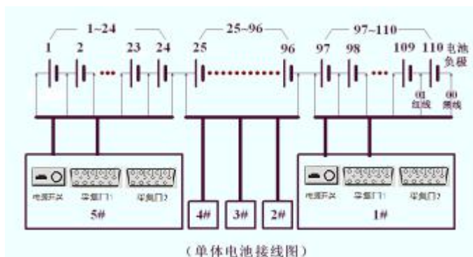
图 2.4.4-3 多个单体模块与电池连接图
