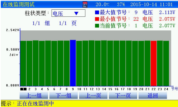
图 3.1.4-1 单体电压柱状图
