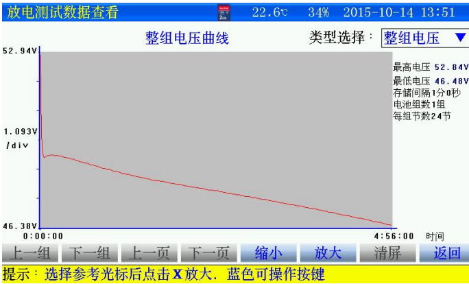
图 3.7.4 整组电压曲线界面
