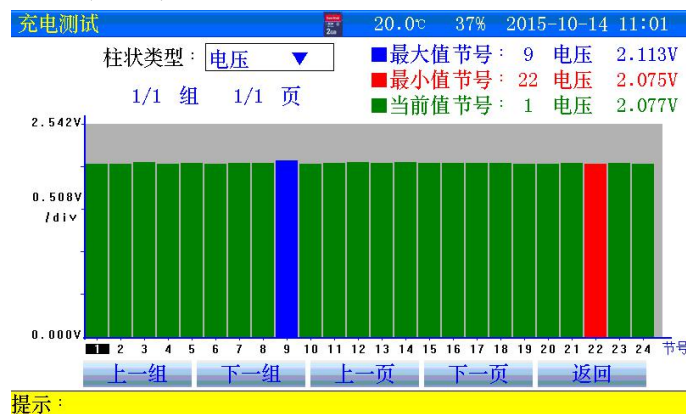
图 3.3.4-1 单体电压柱状图
