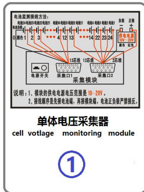
图 2.4.3 单体模块正图
