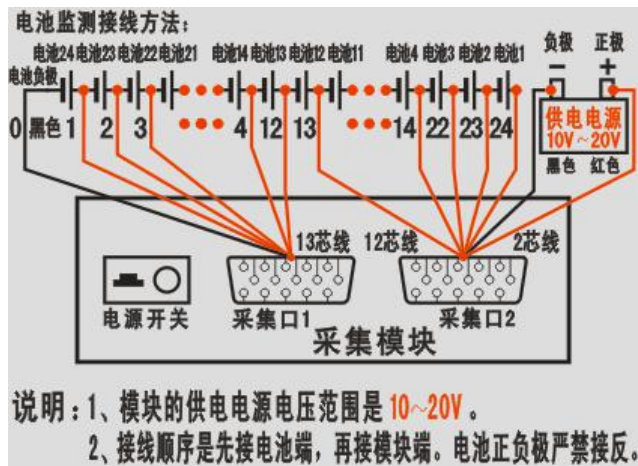
图 2.4.4 24 节 2V 电池与 1 个单体模块连接图
