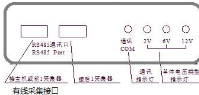
后侧面板图
